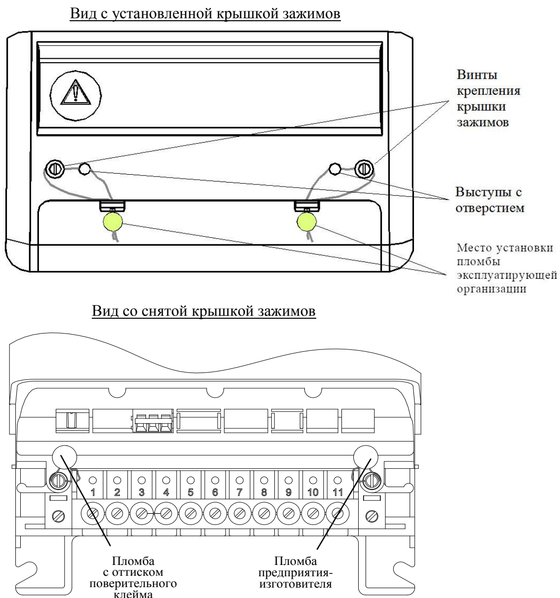
Рисунок 11.1 – Пломбирование счетчика
