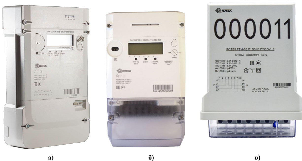
Рисунок 1.1 Основной вид счетчика РТМ-03:
