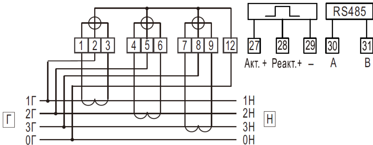
б) Трансформаторное включение (через трансформаторы тока)
