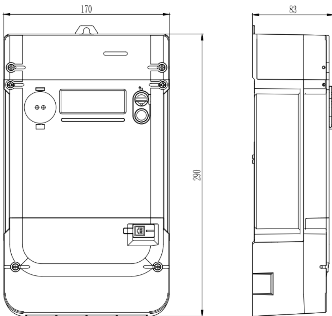
Рисунок 3.4 Размеры счетчика
