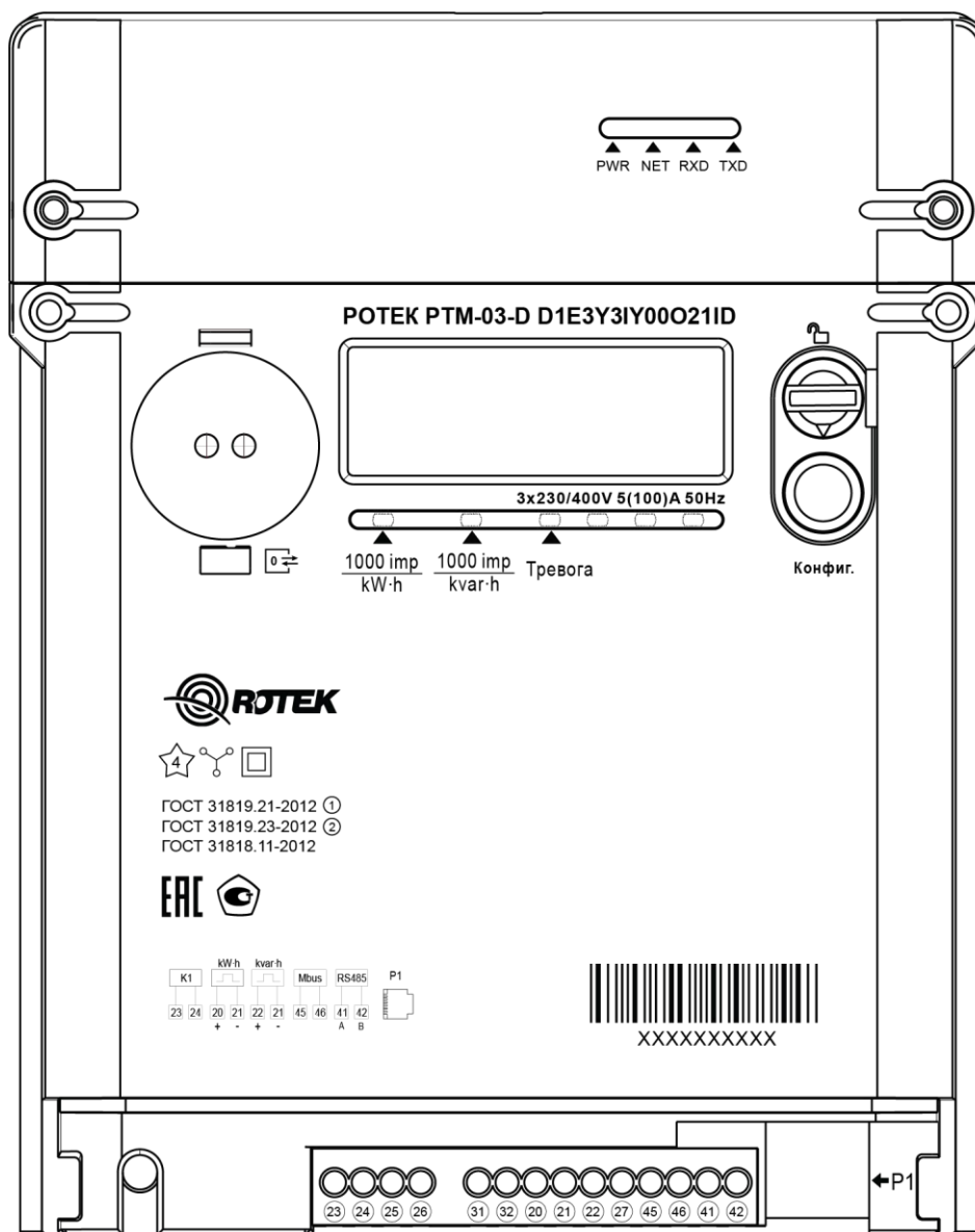
Рисунок 3.2-2. Лицевая панель счетчика РОТЕК PTM-03 трансформаторного включения
