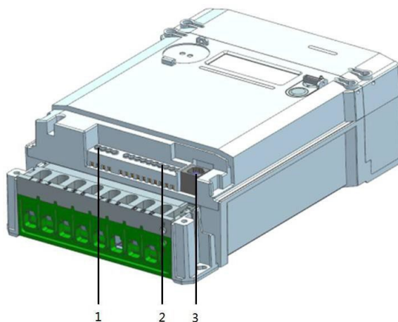
Рисунок 6.4-1 Расположение клемм ввод/вывод для счетчика прямого включения.
