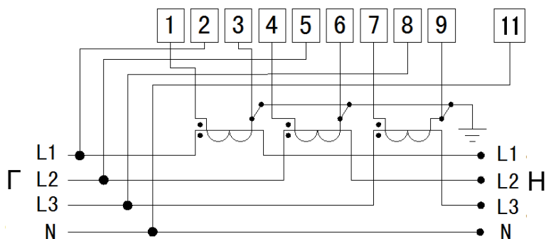
Рисунок 6.1-2 Подключение 3-х фаз и нейтрали для счетчика трансформаторного включения
