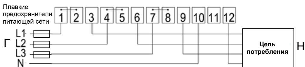
Рисунок 6.1-1 Подключение 3-х фаз и нейтрали для счетчика прямого включения
