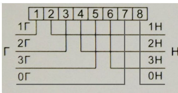
Рисунок 5.3. Диаграмма подключения счетчика к силовой сети
