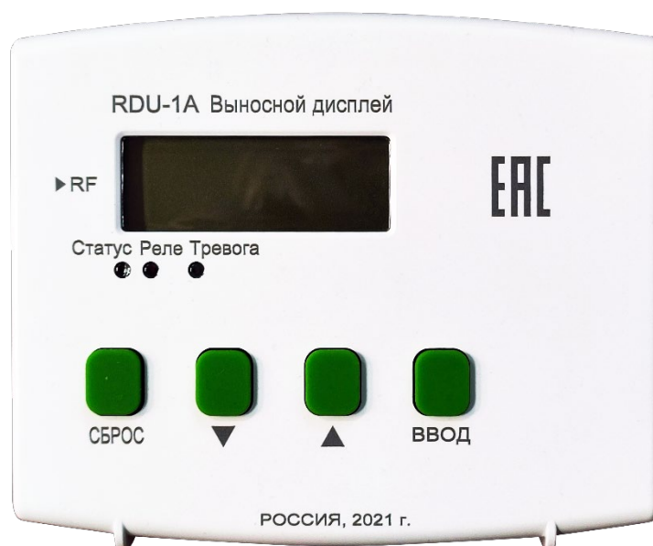
Рисунок 5.4. Внешний вид индикаторного устройства
