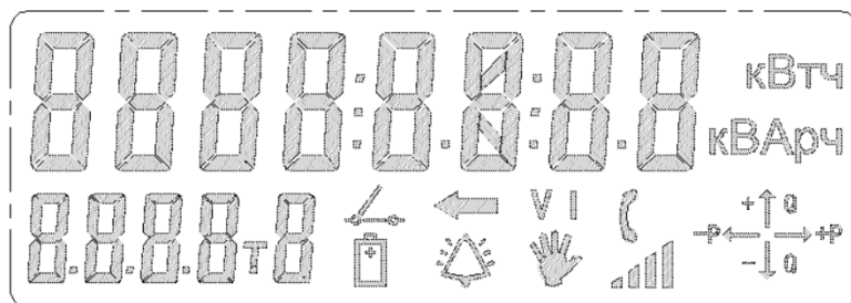
Рис. 5.5 Конструкция индикаторного устройства, LCD дисплей.
