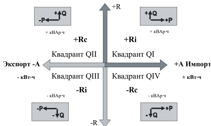
Рисунок 1.3 Четырехквadrантное измерение
