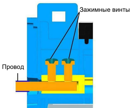
Рисунок 6.3-2 Фазовая клемма
