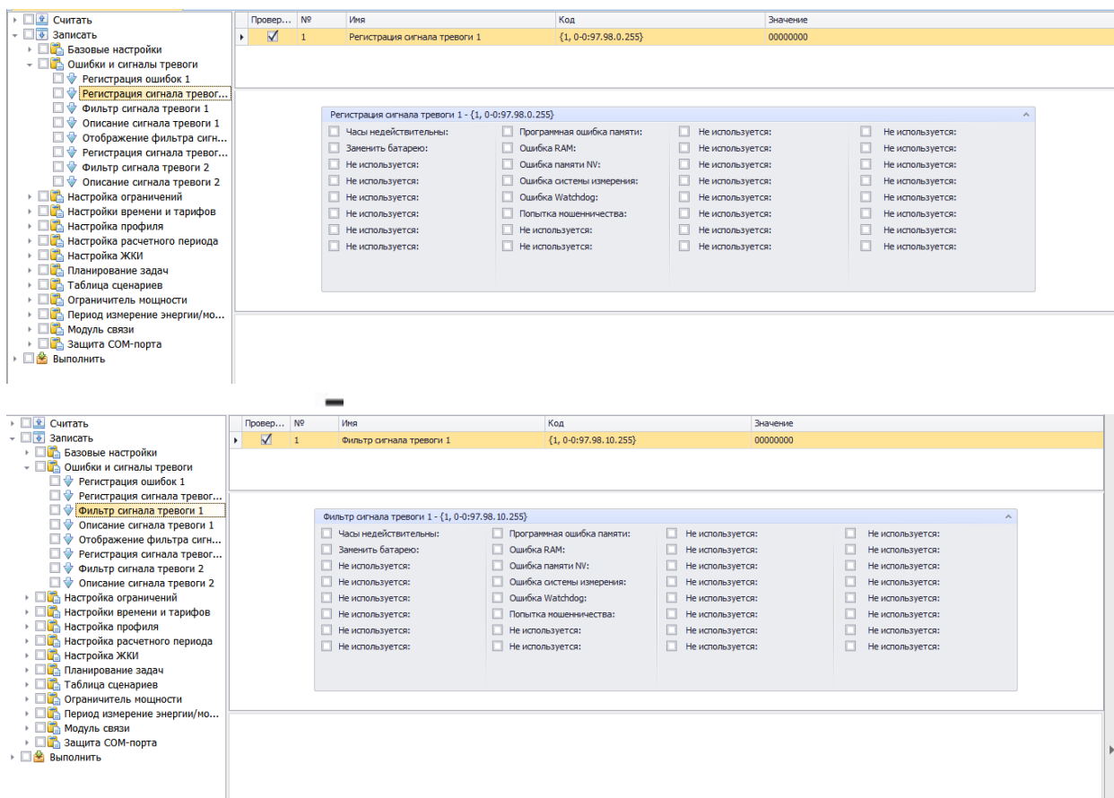
Рисунок 7.5 Конфигурирование параметров инициативного выхода
