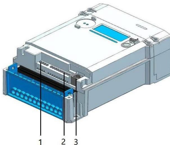
Рисунок 6.4-2 Расположение клемм ввода/вывода для счетчика косвенного включения
