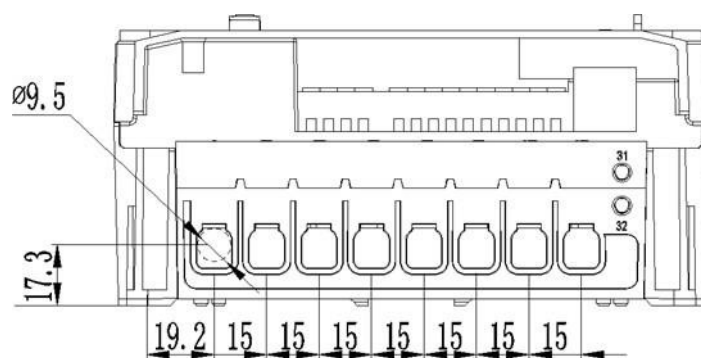
Рисунок 3.5-1 Расположение и размеры клемм для счётчика прямого включения
