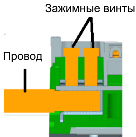
Рисунок 5.3-1 Фазовая клемма
