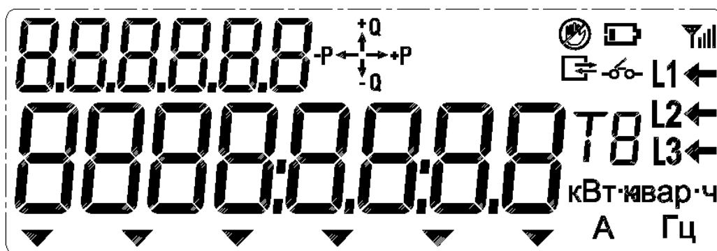
Рисунок 4.2. LCD дисплей.
