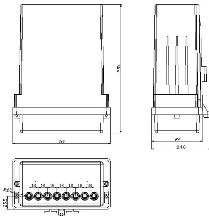
Рисунок 5.7. Размеры счетчика РОТЕК РТМ-03 С
