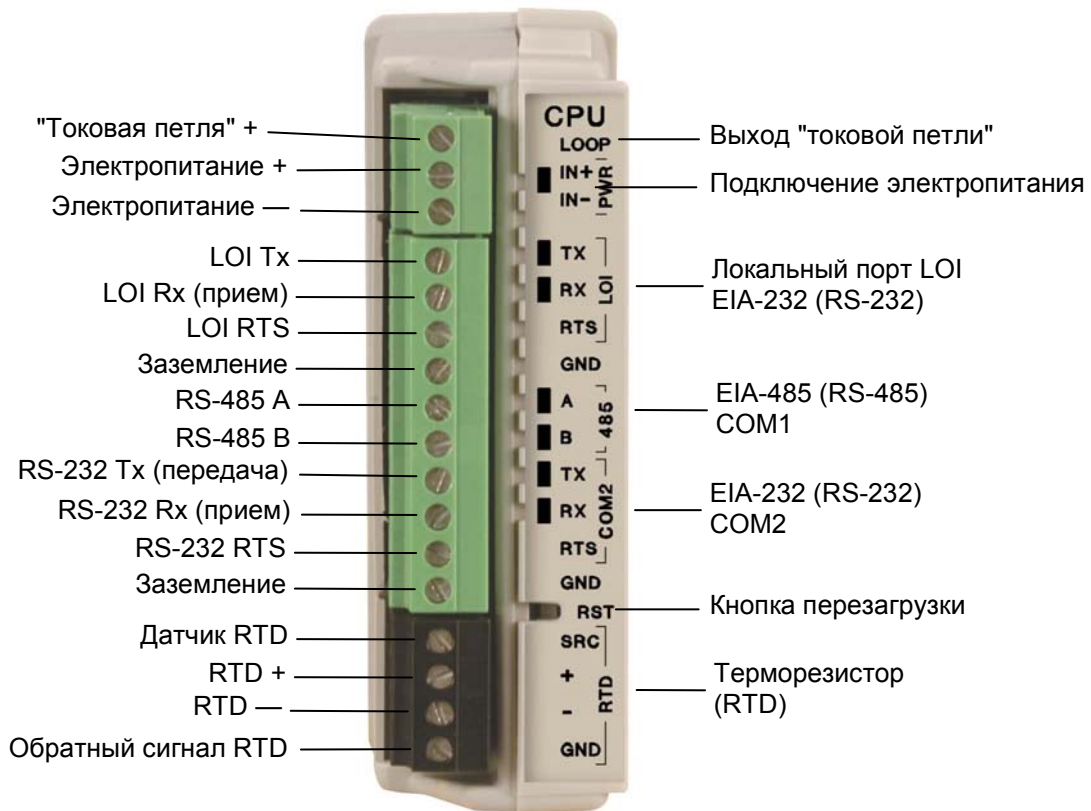
Рис. 2-6. Модуль CPU
