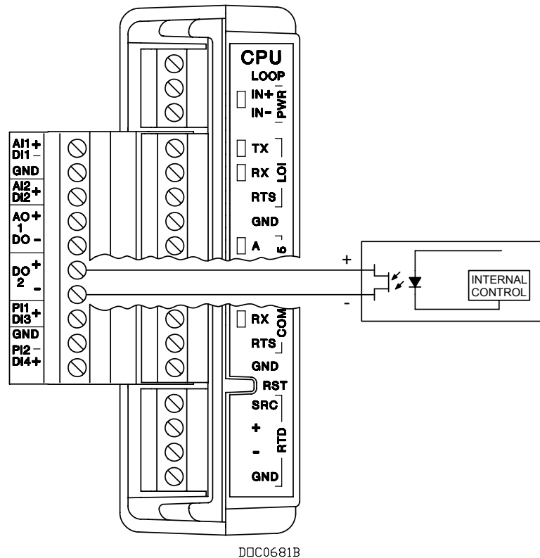
Рис. 4-10. Дискретные выходы
